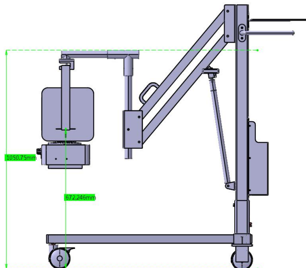
【Figure 2: Lowest extension】
